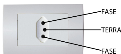
Caso 2: 220 Vca
