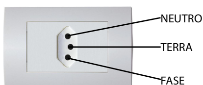
Caso 1: 110 Vca
