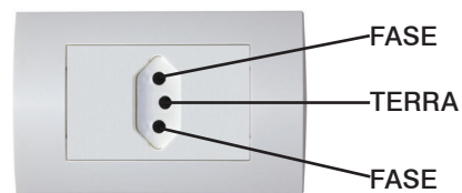
Caso 2: 220 Vca
